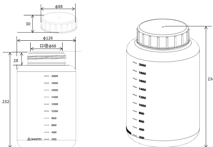
製品外観図
